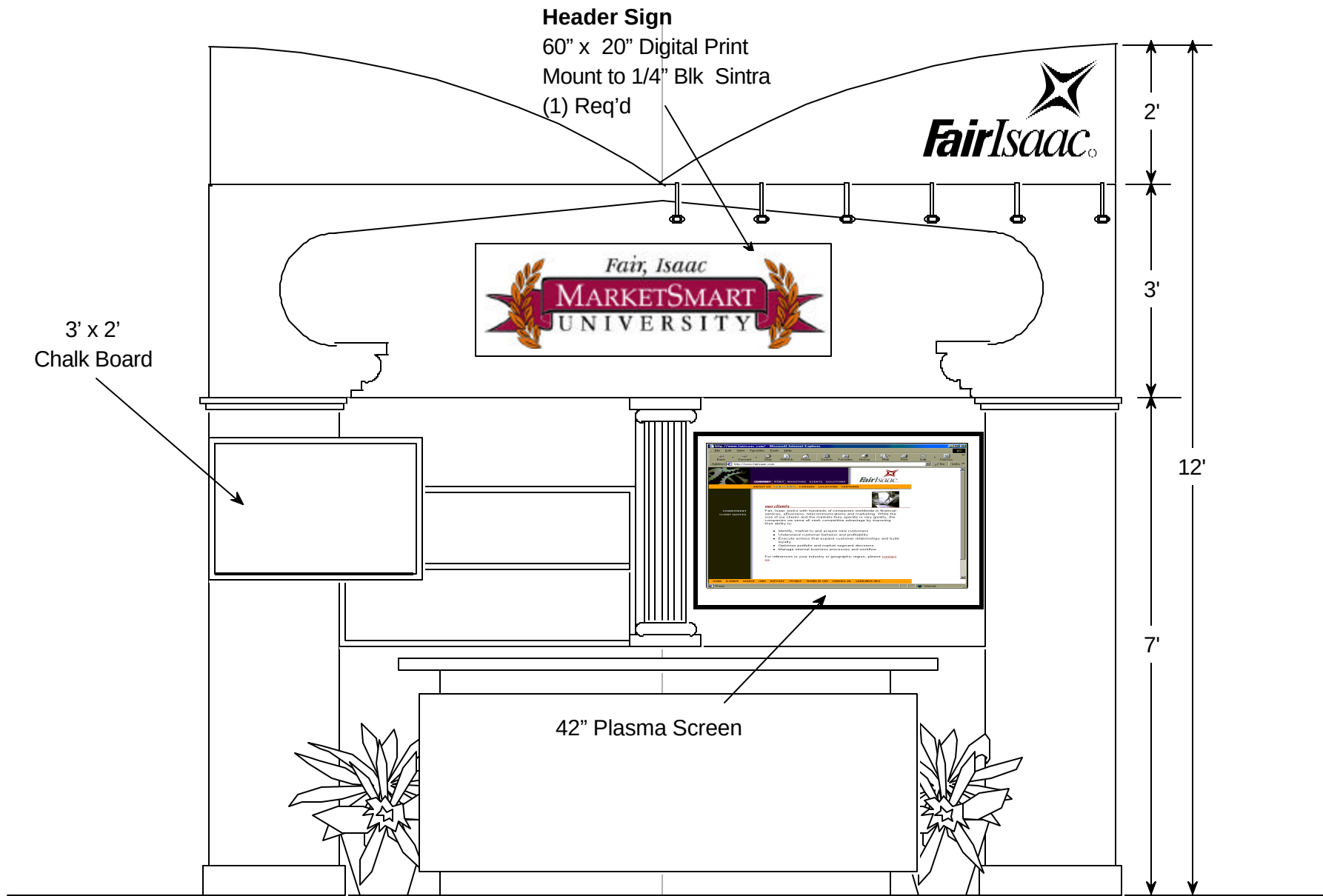
Elevation A
